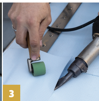
3 Membrane de finition soudée à chaud
