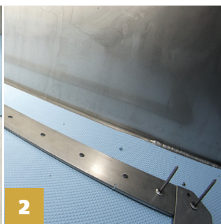
2 Liaison mécanique membrane/inox
